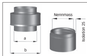
Typ 1 Dila/Stulpring Isolation 25 mm
