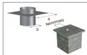
Typ 3 – eckiges Tablett mit rundem Stutzen
