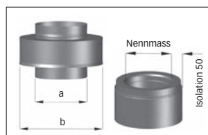
Typ 1 Dila/Stulpring Isolation 50 mm
